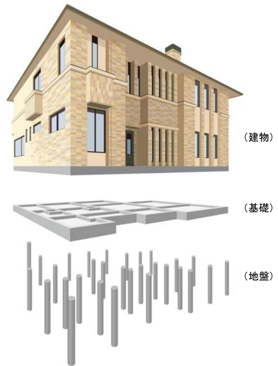
建物・基礎・地盤を一体で計画 (イメージ図)
